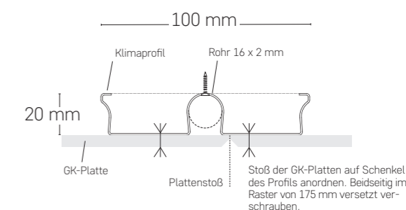
Verschraubung GK-Platte auf Klimaprofil
