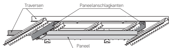
Montage Revisionsklappe
