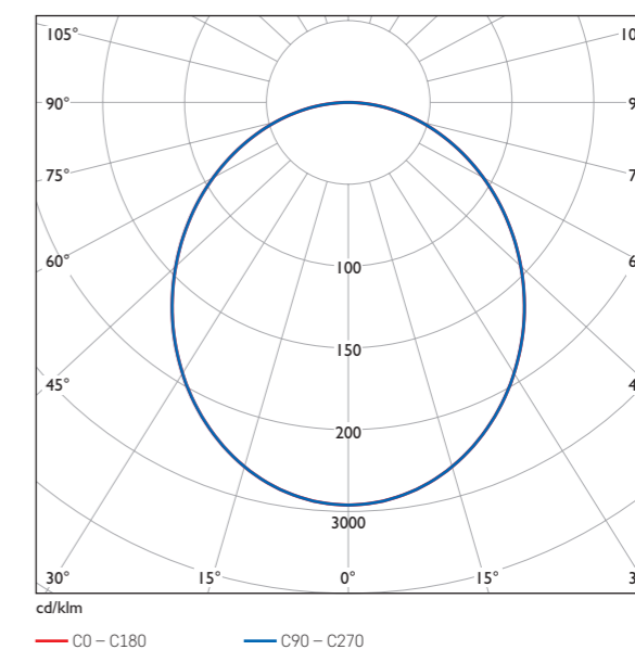
Lichtverteilungskurve Opal
