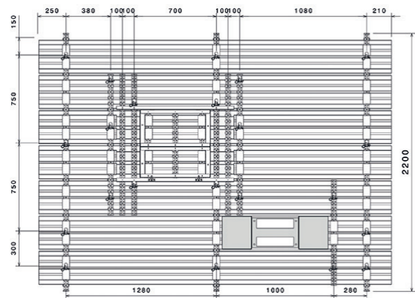
Klimadecke Prüffläche
