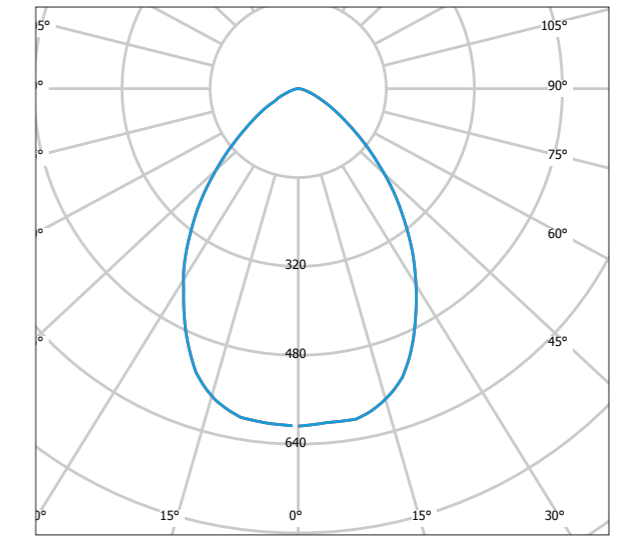
Lichtaustrittswinkel 80°
