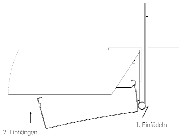
Einclippen Aluminiumpaneel
