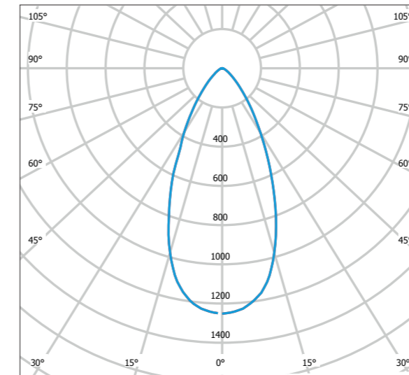
Lichtaustrittswinkel 50°
