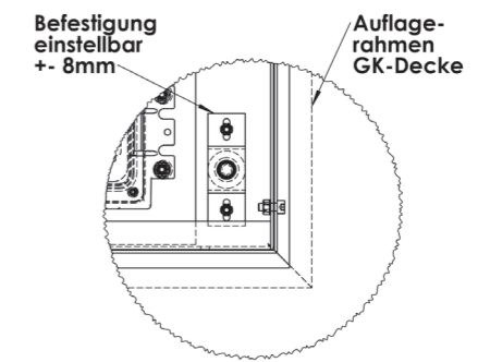
DETAIL Y Maßstab 1 : 2.5
