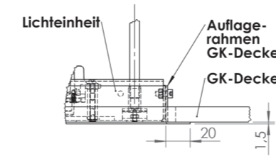
DETAIL X Maßstab 1 : 2.5
