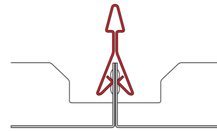
Klemm-Klappsystem
