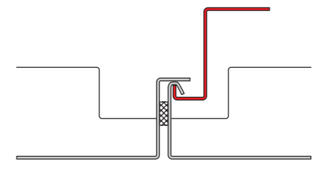
Einhängesystem
