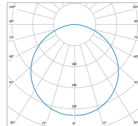
Lichtaustrittswinkel 120°
