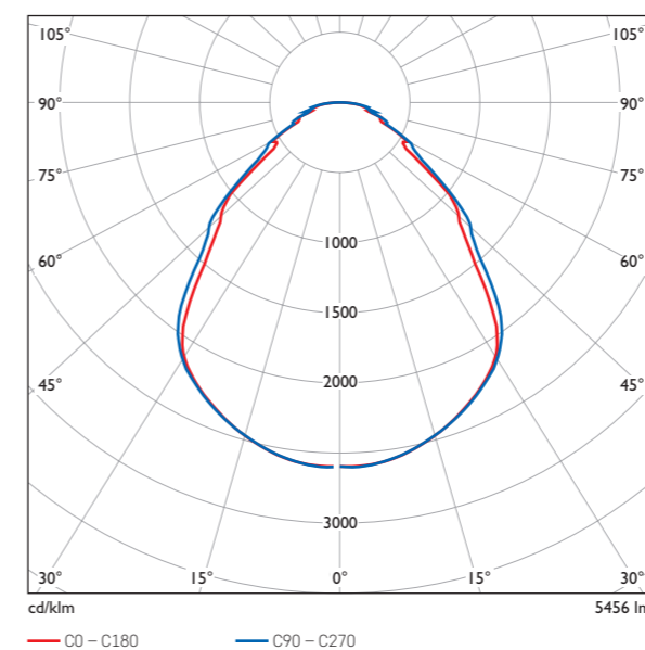
Lichtverteilungskurve Mikroprismen
